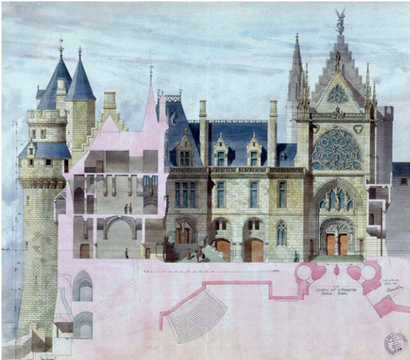
Schloss Pierrefonds Ansicht und Schnitt im Hinblick auf die Erneuerung Aquarell von Viollet-le-Duc, ca. 1857 (Paris, Centre Georges Pompidou)
