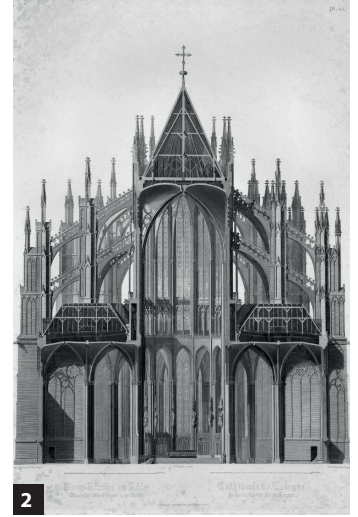
1 Karl Begas d.Ä. (1794-1854), Sulpiz de Boisserée, Bleistiftzeichnung von 1822, Köln Privatbesitz 2 Kölner Dom, Querschnitt durch den Chor in der Breite. aus dem „Domwerk“ von Sulpiz de Boisserée (Zeichnung von Maximilian Heinrich Fuchs 1809, Stich von Christian Friedrich Traugott Duttenhofer 1811/14)
