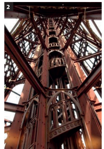
Die gotische Kathedrale von Rouen (F) (1), 12./13. Jh., erhielt erst 1884 einen neuen, sehr hohen Vierungsturmaufsatz (2) aus Eisen und Gusseisen. Formal dem Konformitätsprinzip folgend, materiell und konstruktiv aber zeitgenössisch nach neuestem Stand der Technik
