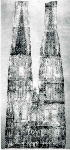
Mittelalterlicher Fassadenplan (Plan F) des Kölner Doms Zeichnung, Feder/auf Papier, um 1300 (Köln, Dombauarchiv)
