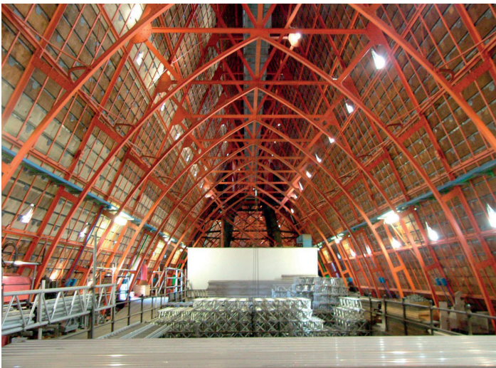
Bei der Vollendung des Kölner Doms hat man sich der neuesten Technik bedient und im Dach keine Holzkonstruktion, sondern ein modernes Eisentragwerk eingebaut.
